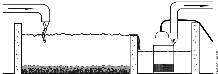
Abbildung 1: Absetzpumpensumpf
